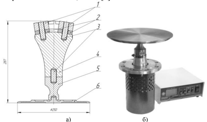
а – конструктивная схема; б – внешний вид 1 – задние отражающие накладки, 2 – пьезоэлектрические элементы, 3 – стягивающие шпильки, 4 – преобразователь, 5 – концентратор, 6 – дисковый излучатель
